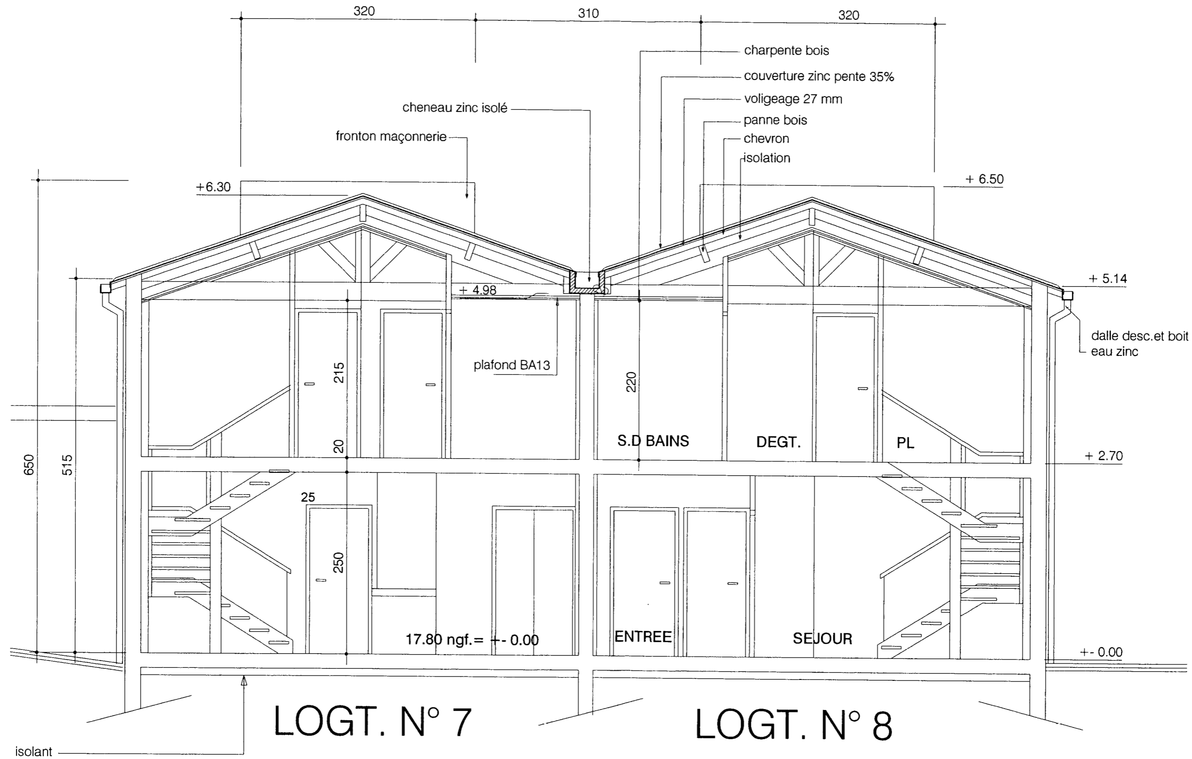
Coupe 1-1
