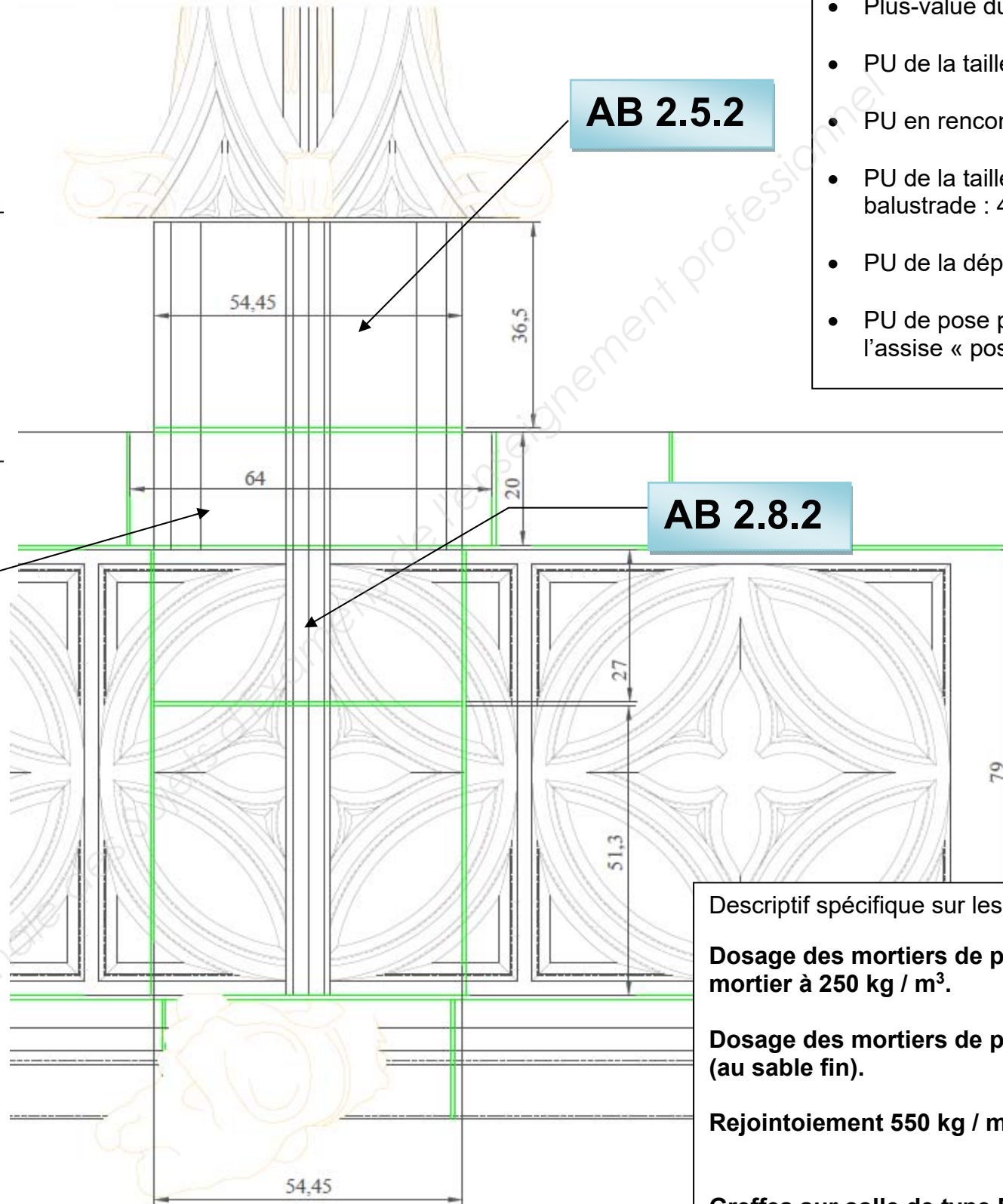
Élévation
