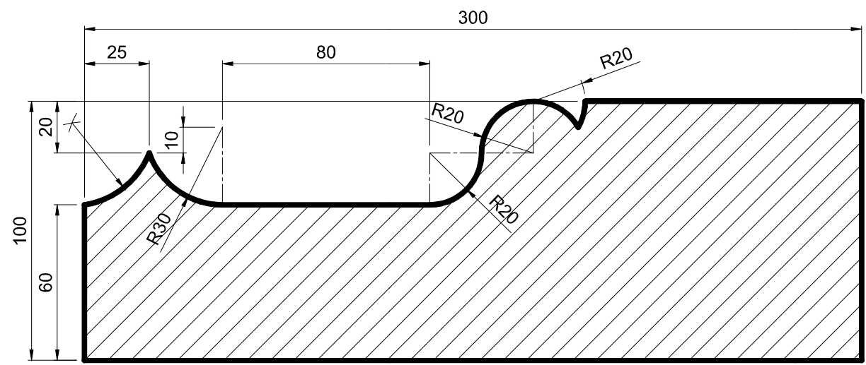
Profil de moulure
